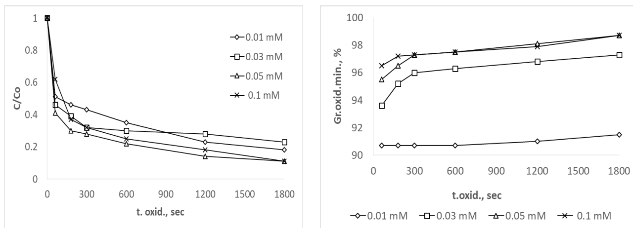
Figura 3. Influența concentrației catalizatorului asupra gradului de oxidare (b) și de degradare (a) a AMX; [AMX]_0=200 mg/L, [H_2O_2]_0=3 mM, pH= 2,2, T= 25° C.
